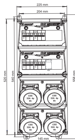
PLANO MECÁNICO
