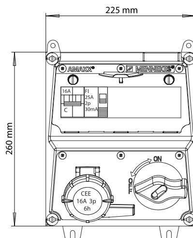
PLANO MECÁNICO
